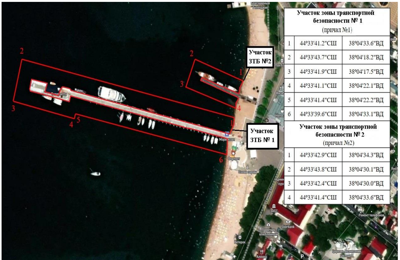
Схема Участка №1 и Участка №2 ЗТБ ОТИ «Акватория морского порта Геленджик»
